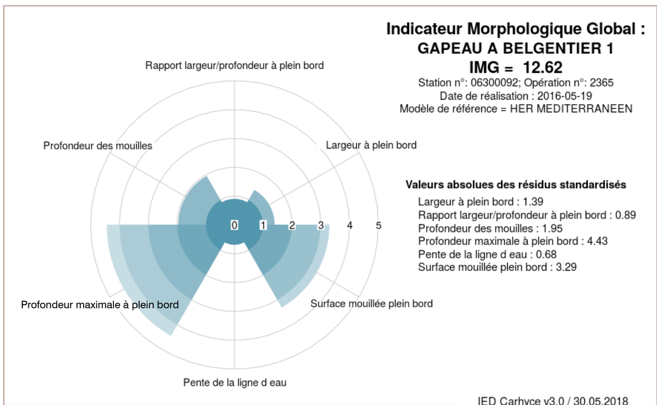
Figure 45 - Représentations graphiques de l'Indicateur morphologique global (IMG) de deux opérations : le Tarn à Montbrun (2011) et le Gapeau à Belgentier (2016) [30]. Plus la projection sur les axes est réduite et centrée sur 0 (zéro), plus l'indicateur est faible pour les 6 paramètres qui le composent ; alors la situation supposée de la station est proche des tendances naturelles (sans ou avec peu de pressions liées aux activités humaines) régionales.
