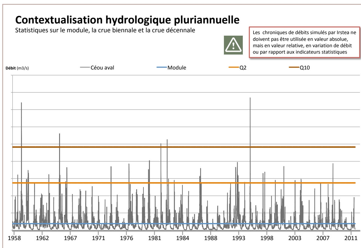
Figure 62 - Exemple de chronique hydrologique pluriannuelle sur le Céou aval (source des données : reconstitution de chroniques hydrologiques Irstea sur le site du projet Carmen http://carmen.carmencarto.fr/66/AFB_Reconstitution-chroniques-hydrologiques.map )
